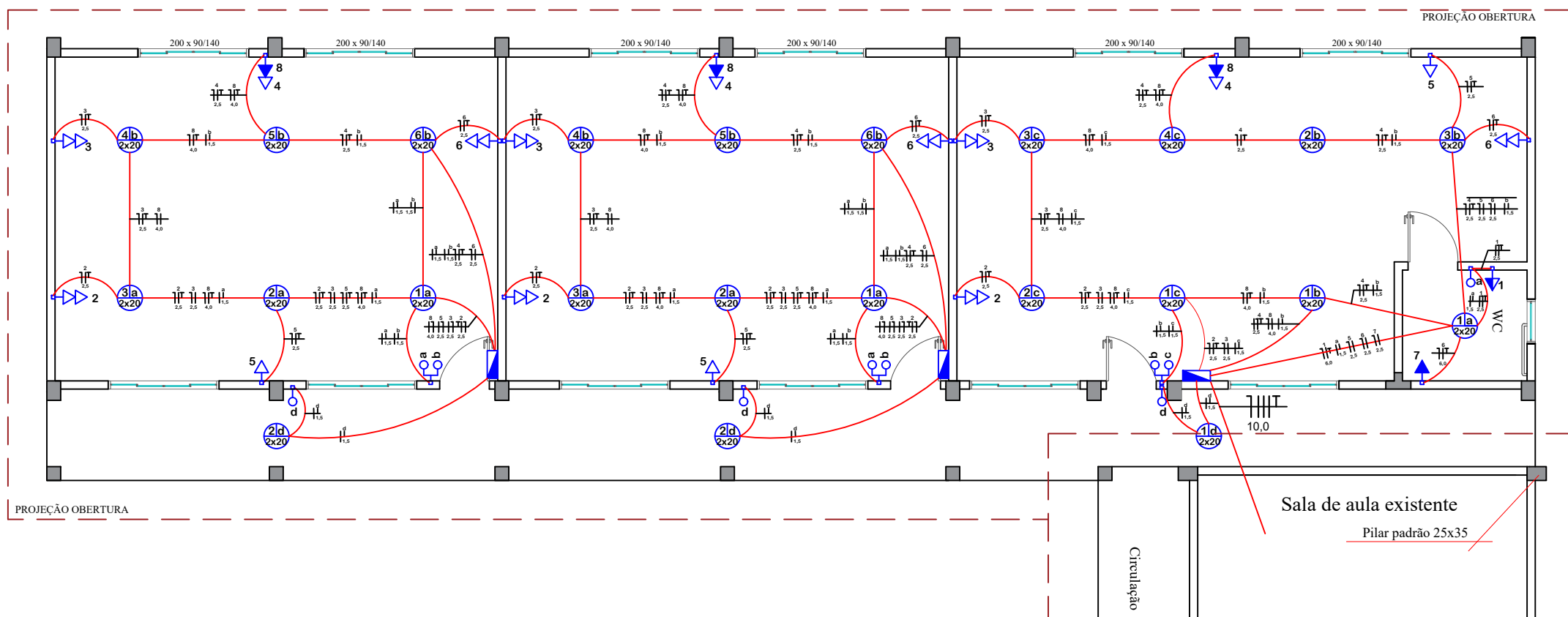
PLANTA BAIXA ELÉTRICO ÁREA CONSTRUÍDA: 199,24 m²
