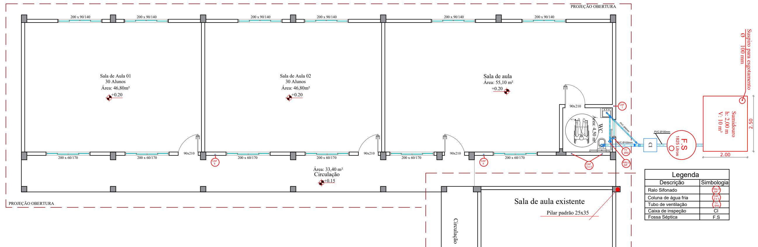
PLANTA BAIXA HIDROSSANITÁRIO ÁREA CONSTRUÍDA: 199,24 m²
