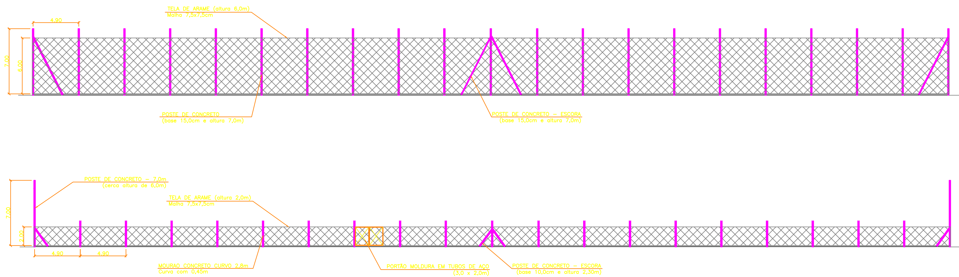
VISTA LATERAL E TARDOZ - ALAMBRADO esc 1:250
